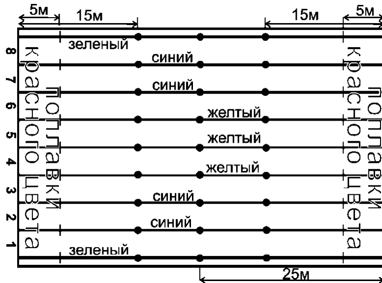
Рисунок 2. Схема расположения разделительных дорожек
