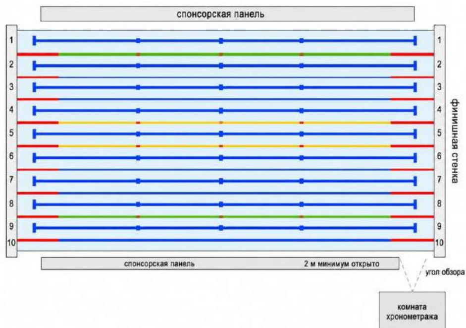
Рисунок 4. Схема размещения спонсорских панелей и светодиодных экранов в чаше бассейна.
