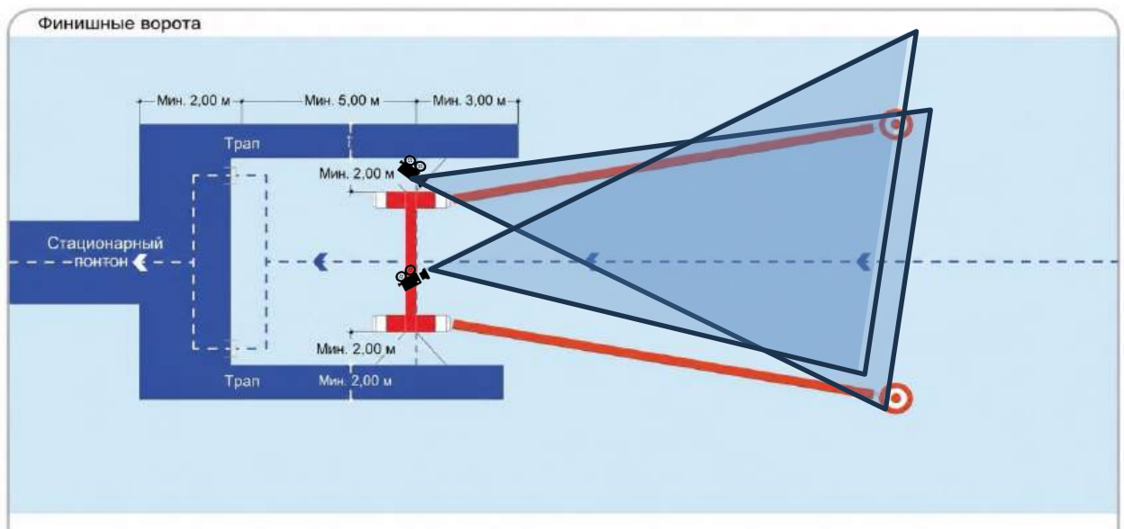
Рисунок 5. Схема обзора видеокамер видеоконтроля на финише
