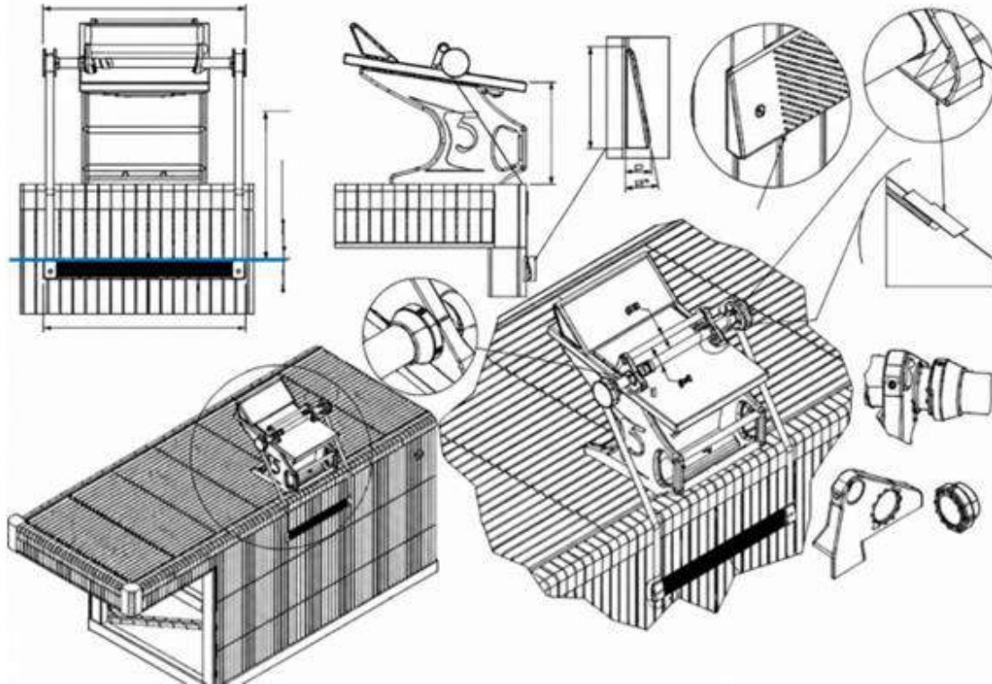
Рисунок 3. Стартовые тумбочки и устройство для старта на спине.
